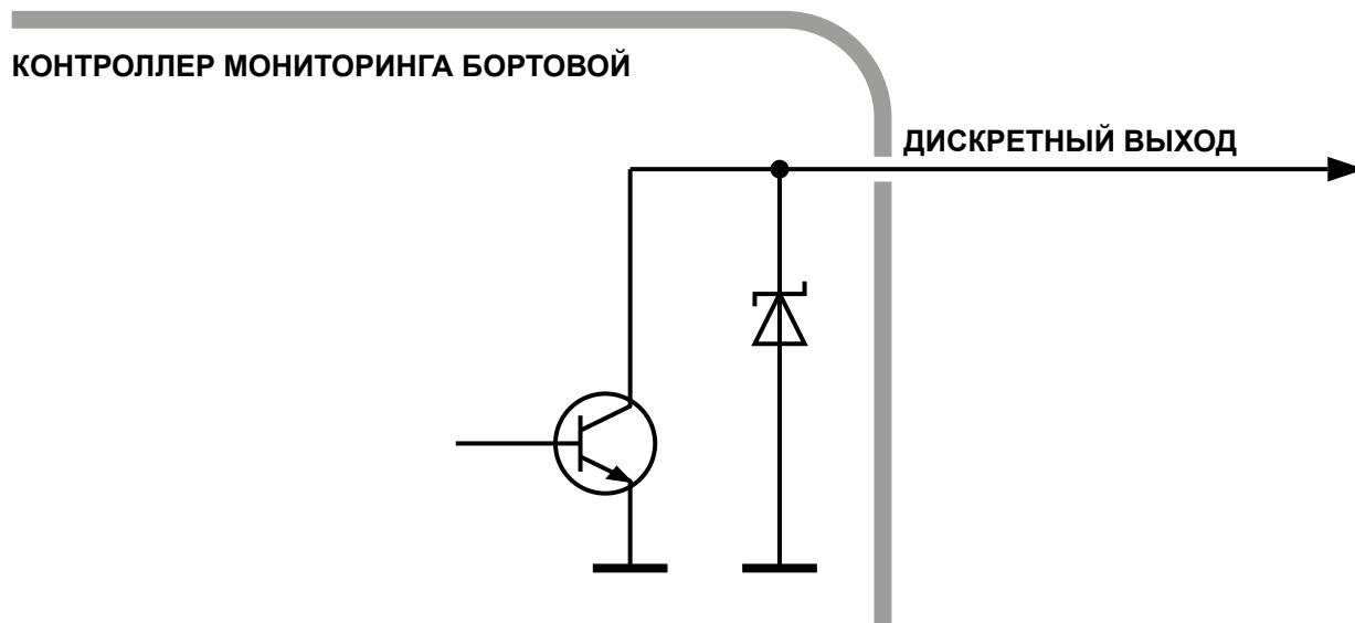
Рис.14. Внутренняя схема выхода.
