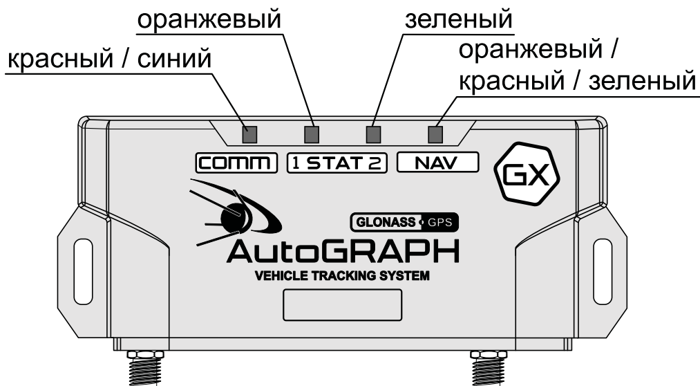
Рис.6. Индикация контроллера.
