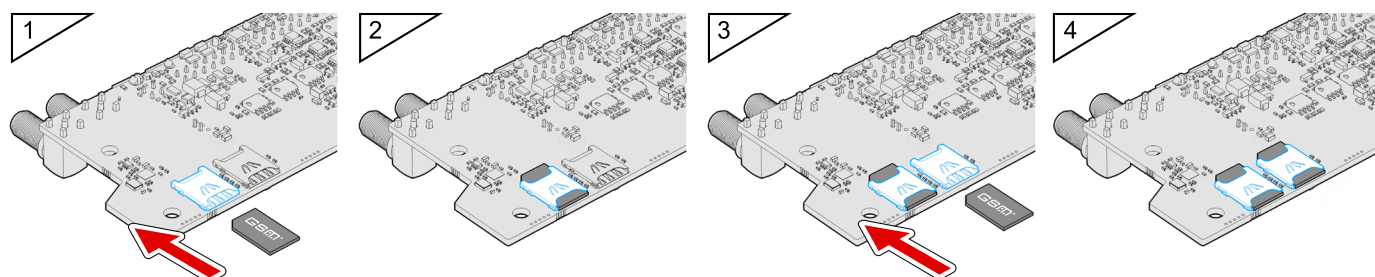
Рис.2. Установка SIM-карты.
