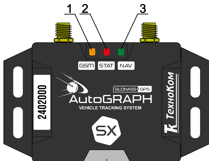
Рис.7. Индикация контроллера.
